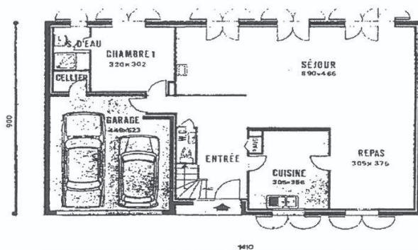
REZ-DE-CHAUSSEE
